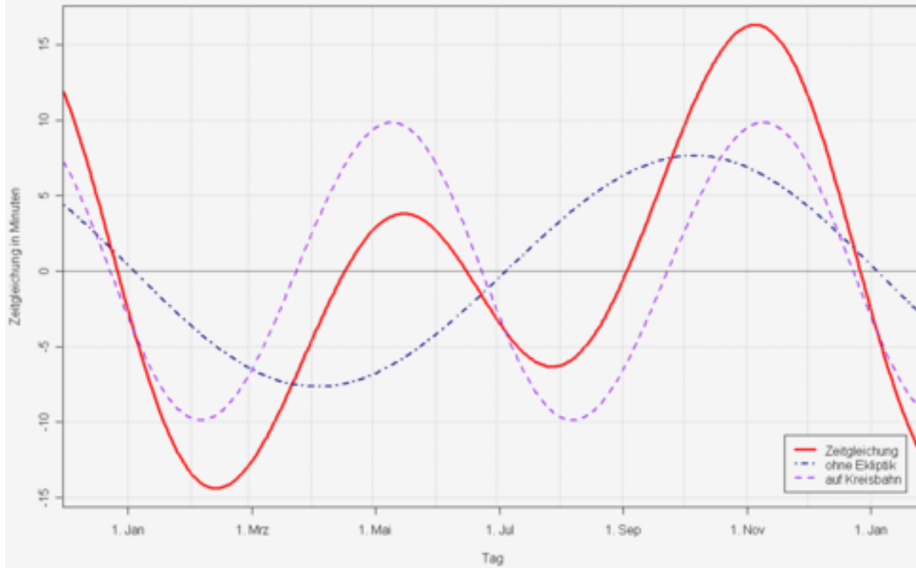
Zeitgleichung: wahre Ortszeit - mittlere Ortszeit
